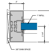
⑦ JAMB 6" = 1'-0"
