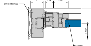
⑪ JAMB Ø = 1'-0"
