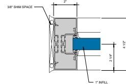
⑩ JAMB 6" = 1'-0"
