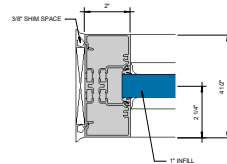
⑩ JAMB 6" = 1'-0"
