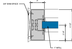
⑩ JAMB Ø = 1'-0"
