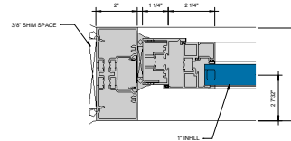
11 JAMB 6" = 1'-0"
