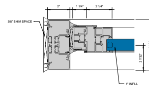
⑪ JAMB Ø = 1'-0"
