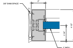
10 JAMB 6" = 1'-0"
